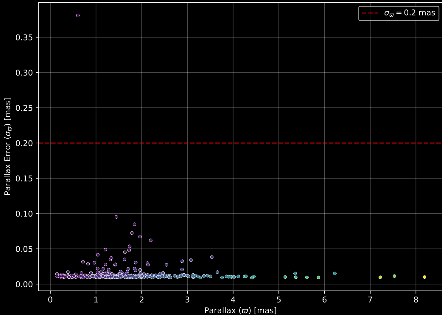
GALAH DR4 Field: [370] Parallax Quality (n= 311)
