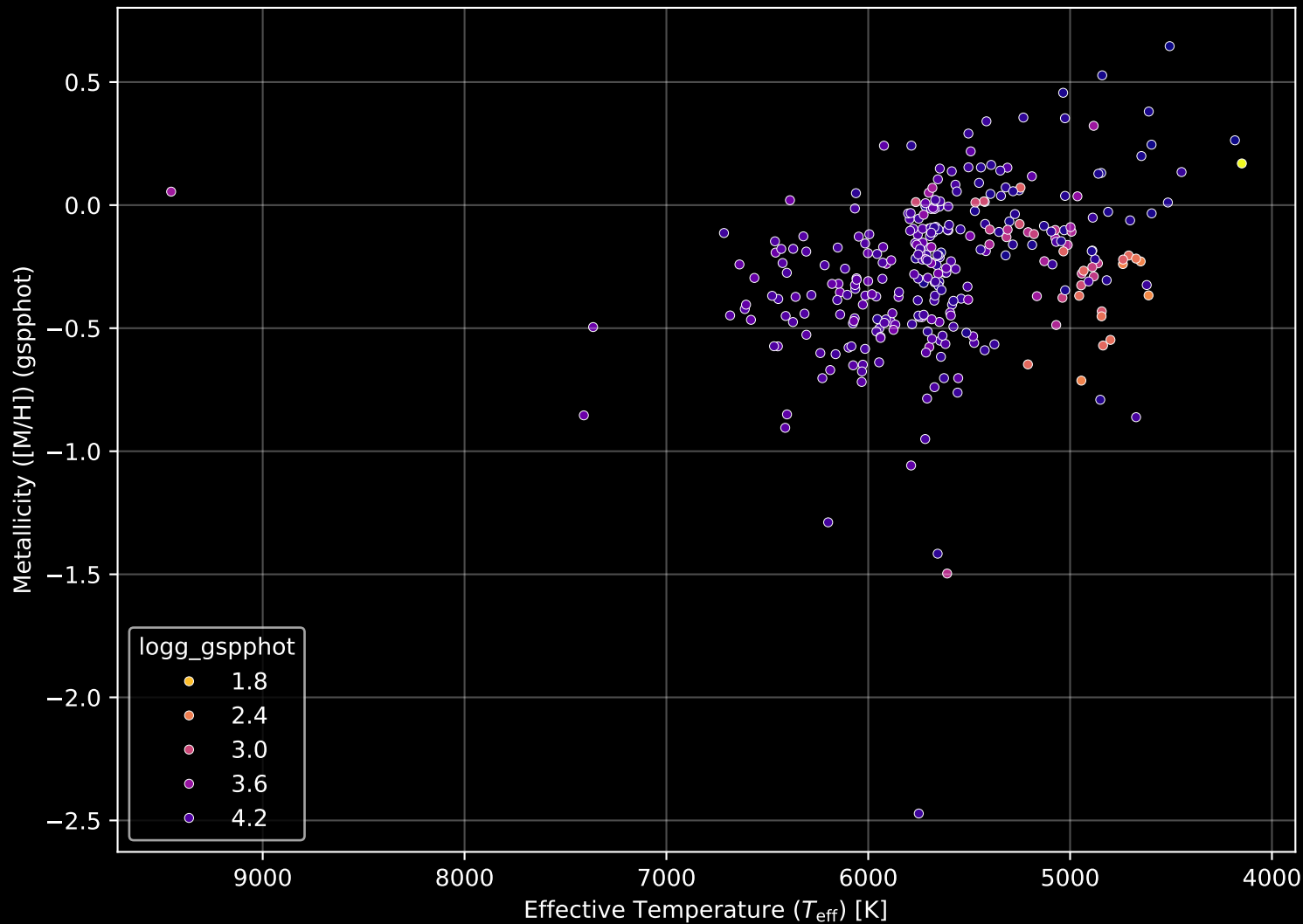
GALAH DR4 Field: [370] Stellar Population Parameters (n= 311)
