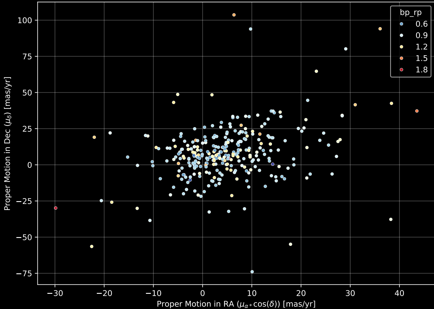
GALAH DR4 Field: [370] Proper Motion Diagram (n= 311)
